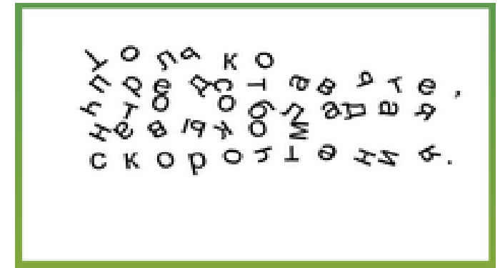
Вращающийся текст
