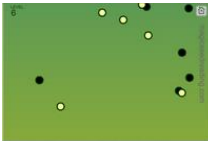
Деконцентрация
